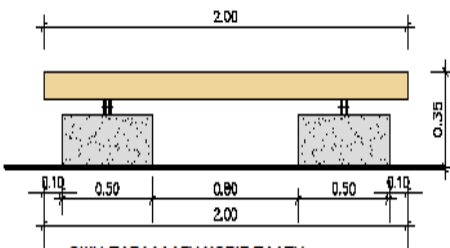
ΟΨΗ-ΠΑΡΑΛΛΗΛΗ ΧΩΡΙΣ ΠΛΑΤΗ
