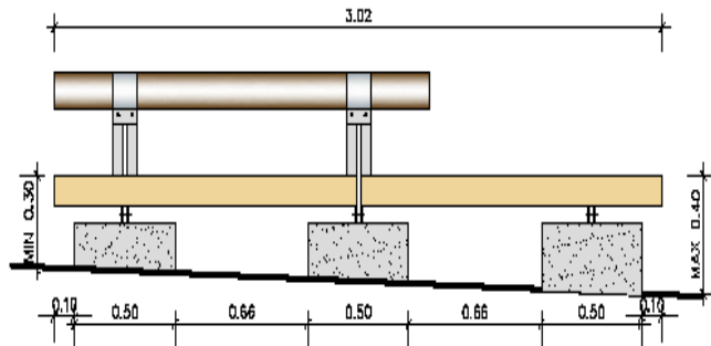
ΟΨΗ-ΠΑΡΑΛΛΗΛΗ ΣΕ ΚΕΚΛΙΜΕΝΟ ΕΠΙΠΕΔΟ
